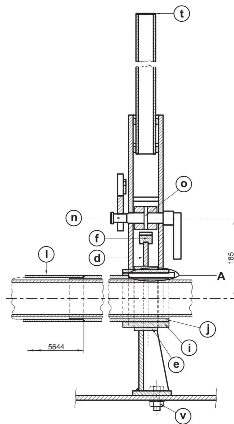
CORTE AA (S/Escala)
