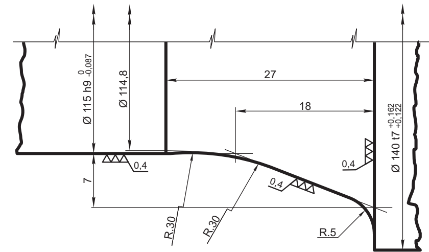
DETALLE D (Esc. 2:1)
