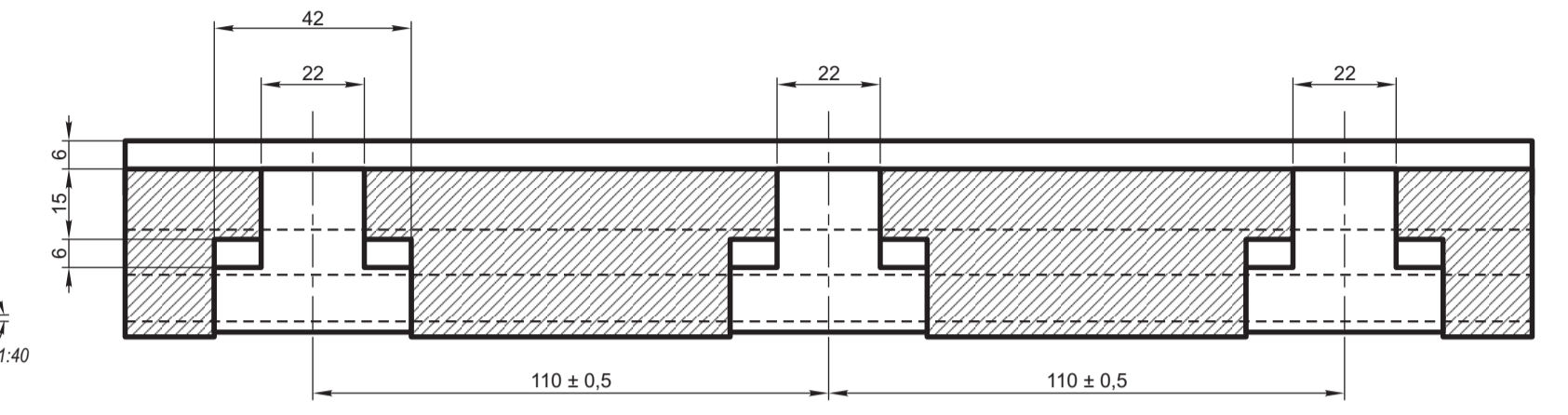
CORTE B-B
