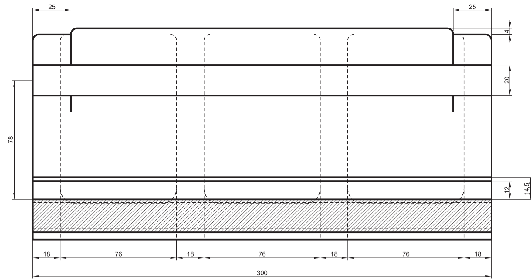
CORTE C-C
