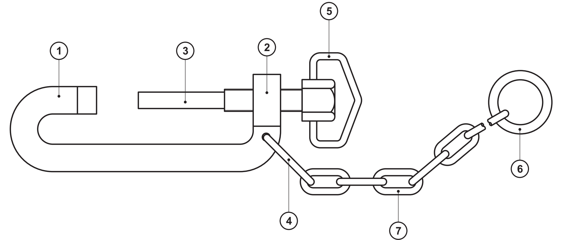
CONJUNTO Es. 1:2,5
