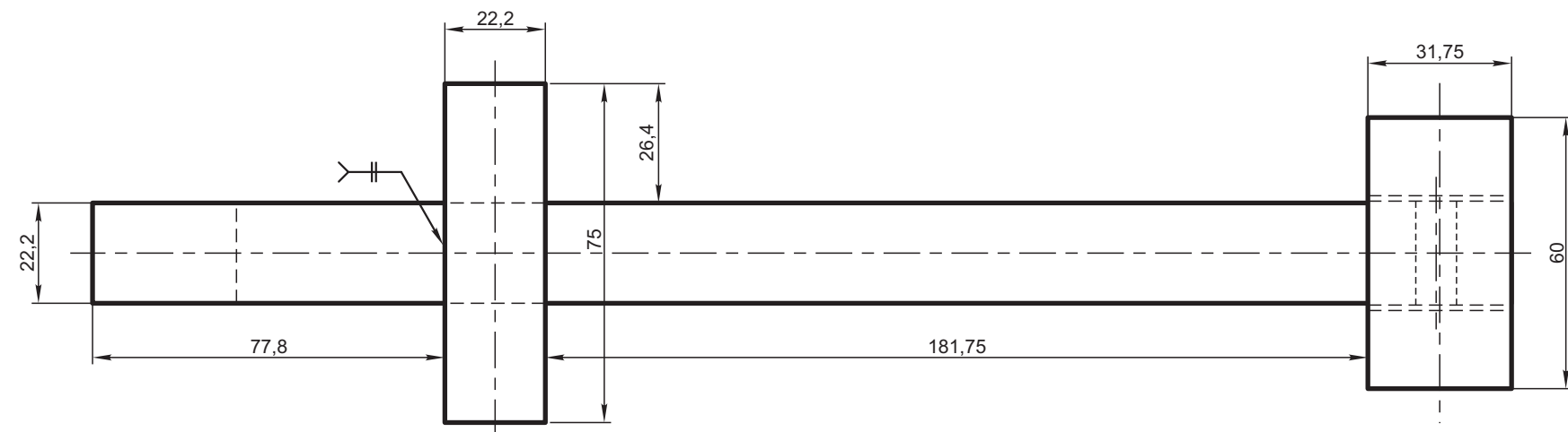
DETALLE PIEZAS 1 Y 2
