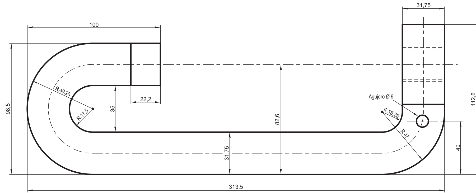
DETALLE PIEZAS 1 Y 2
