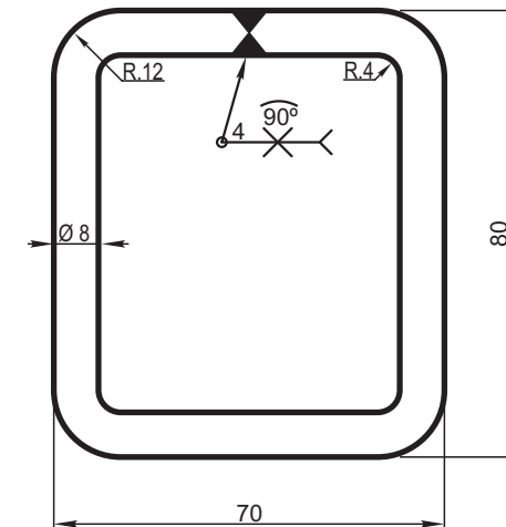
DETALLE PIEZA 4
