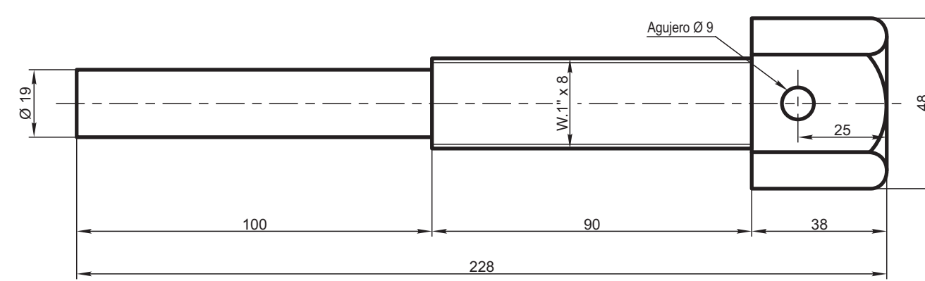
DETALLE PIEZA 3
