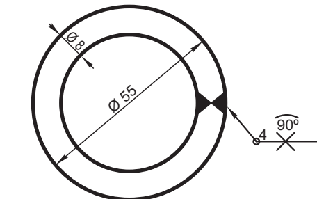
DETALLE PIEZA 6
