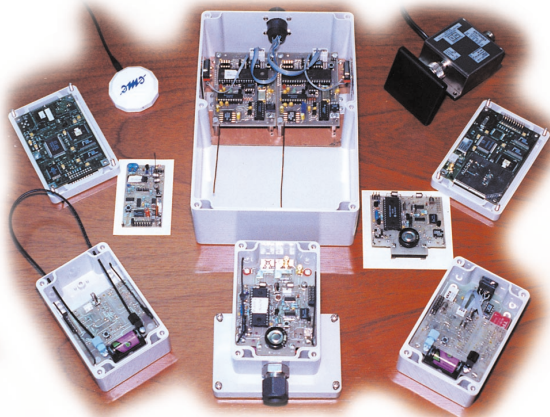
Sensores desarrollados para el sistema de monitoreo remoto
