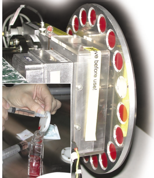
Irradiación de muestras de sangre con partículas alfa en acelerador de iones
