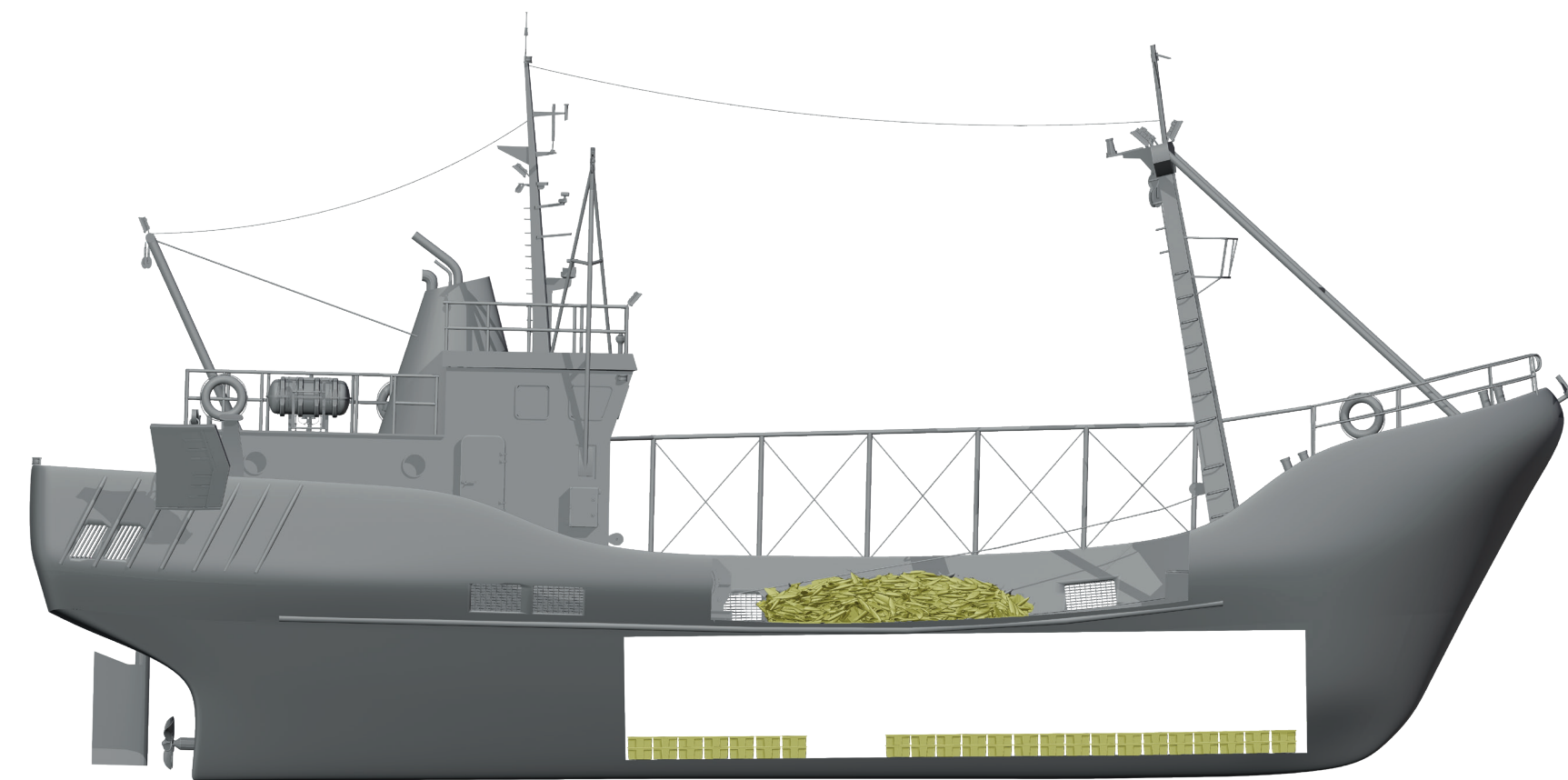
Bodega con poca carga y captura normal en cubierta
