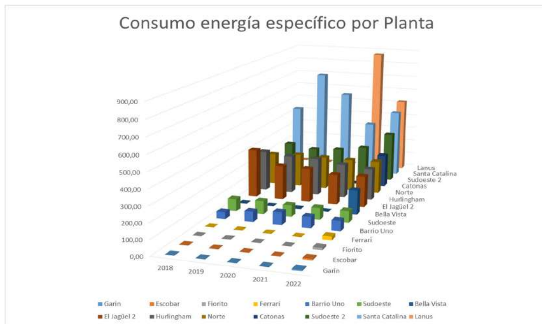
Consumos eléctricos específicos en kW/m³/h
