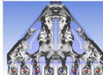
Formaciones Vórticiales
