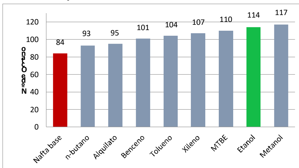
FG166: Mejoradores octánicos utilizados en la formulación de naftas
