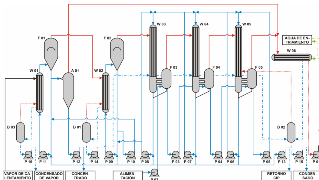
FG143: Esquema funcional de una planta de concentración de vinaza de múltiple efecto
