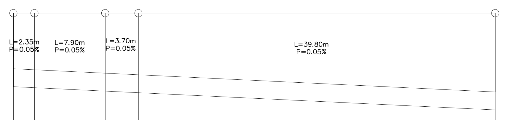
PERFIL LONGITUDINAL DEL COLECTOR PRINCIPAL Escala Horizontal 1:250 Tubería de PVC PN6 DN200mm Velocidad = 0.96 l/s Capacidad a sección llena = 30.13 l/s
