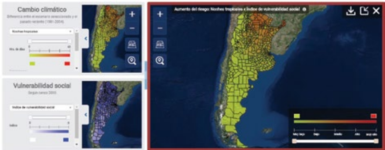
Figura 10. Sistema de Mapas de Riesgo del Cambio Climático.
