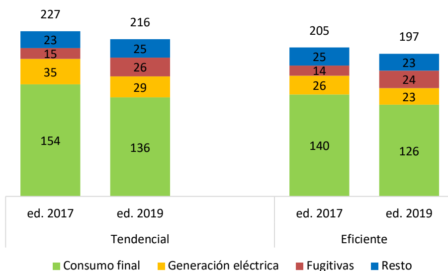
Gráfico: Emisiones vinculadas al sector energético en 2030 según las ediciones 2017 y 2019 de los escenarios energéticos, en MtCO 2 eq
