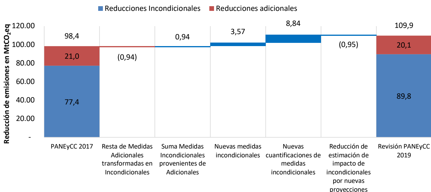
Gráfico: Diferencias en la reducción de emisiones entre el PANeyCC 2017 y su actualización
