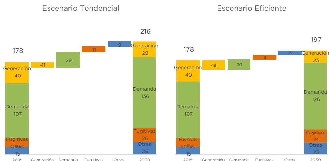
Gráfico: Emisiones de GEI vinculadas al sector energético
