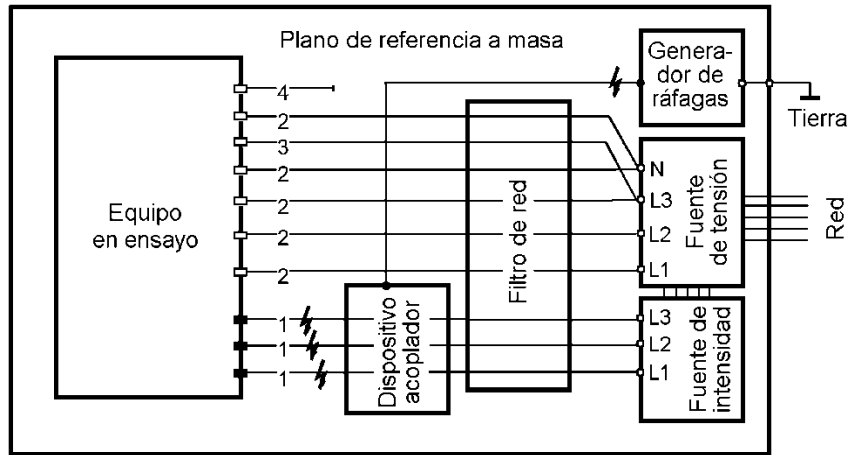
Fig. D.2 – Montaje para el ensayo a los transitorios rápidos en ráfagas: circuitos de tensión
