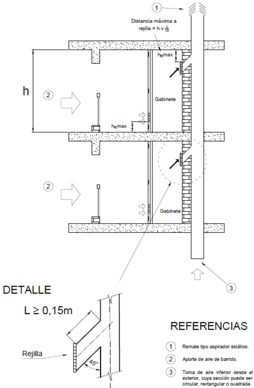
Figura 3.4 - Sala de medidores por piso en pasillos ventilados
