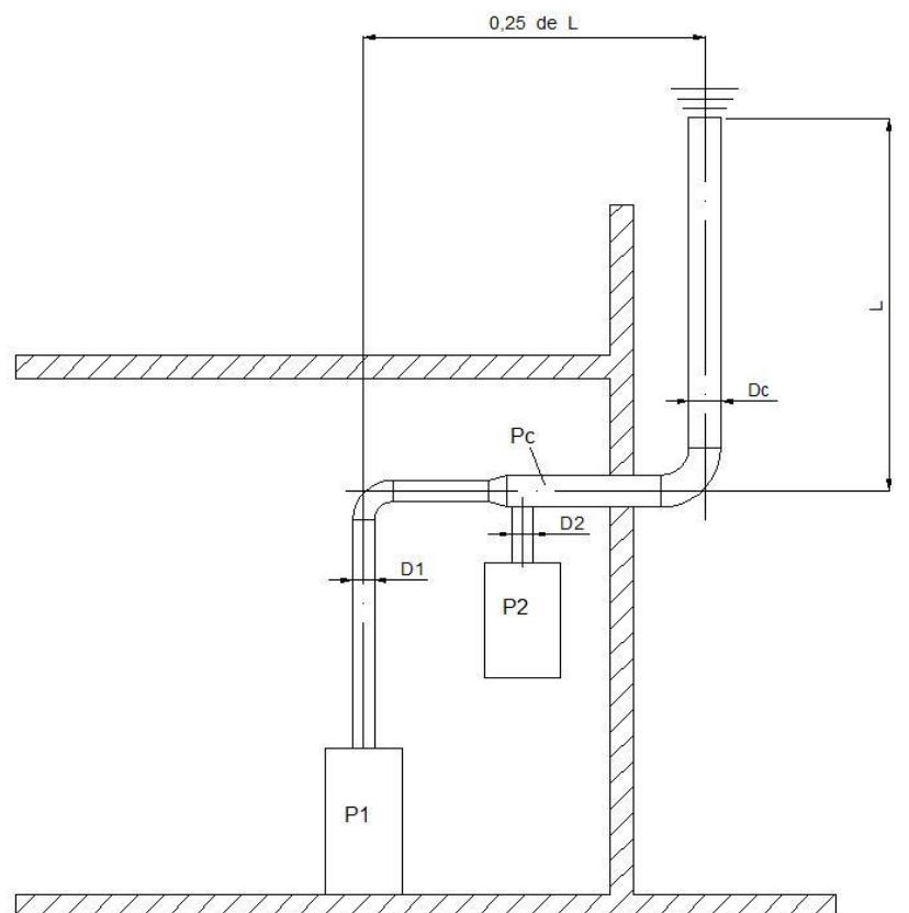
Figura 6.17 a). Colector con desplazamiento lateral
