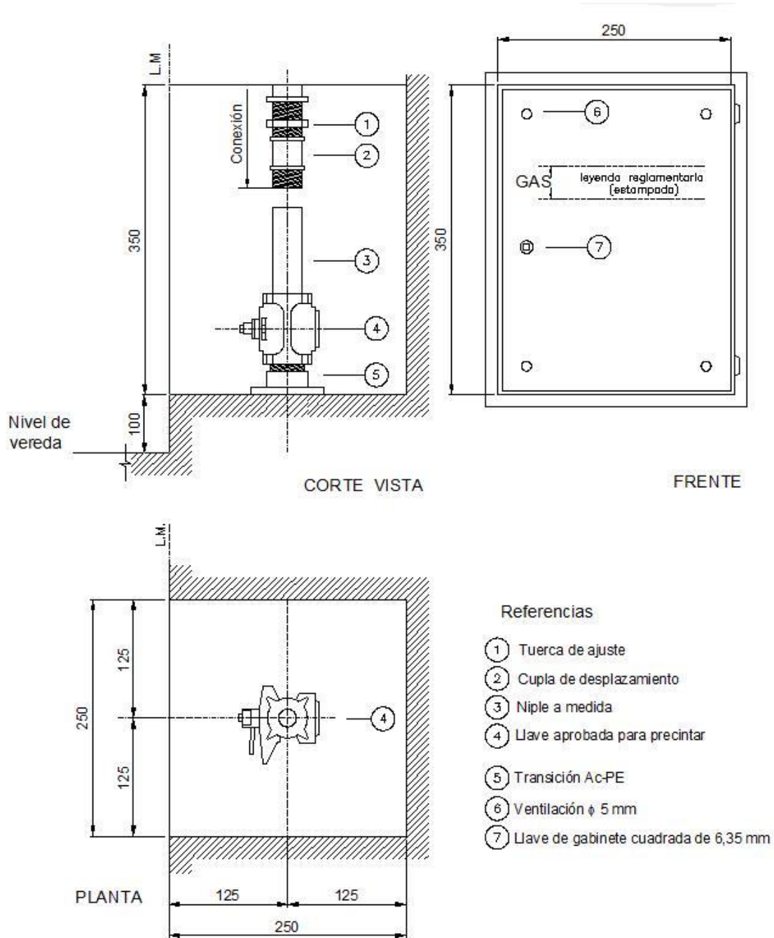
Figura 2.6 - Válvula de bloqueo para medición interna
